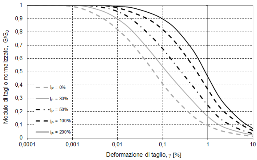
Figura 5 – Curve G/G_0 - \gamma di letteratura per terreni a grana fine (AGI, 2005)
